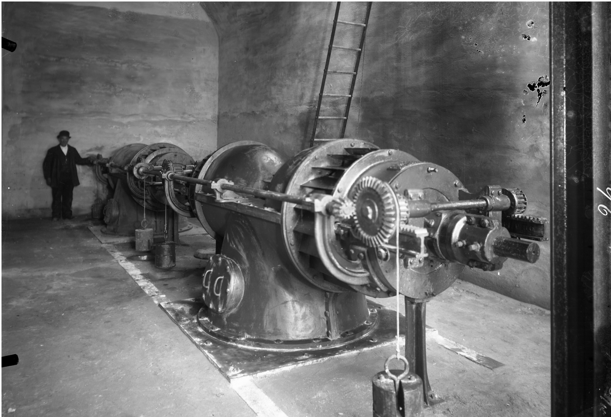
Mann fotografert attmed ei maskin kring 1900. Foto: Ragnvald Nyblin / Telemark Museum.
